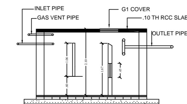
SECTION (N.T.S.)
