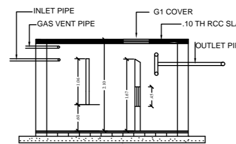
SECTION (N.T.S)
