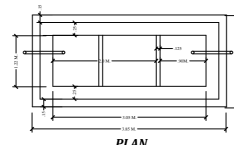
PLAN (N.T.S) DETAIL OF SEPTIC TANK
