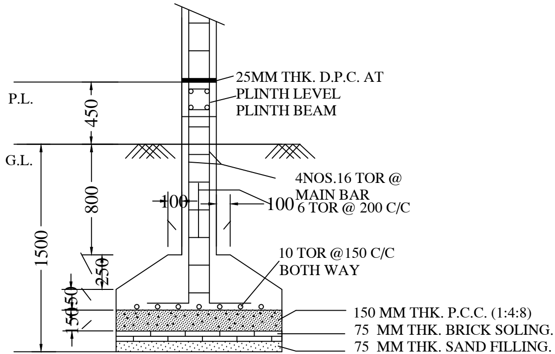
SECTION -CC
