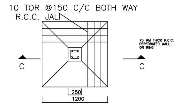
PLAN SCALE:- 1:50
