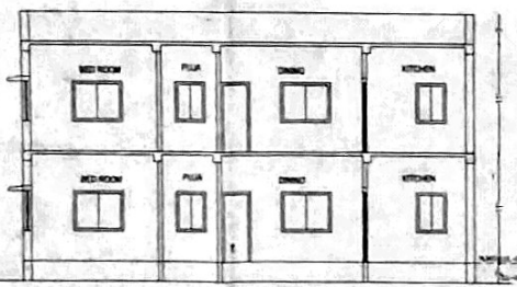
SECTION AT Y Y SCALE 1:100
