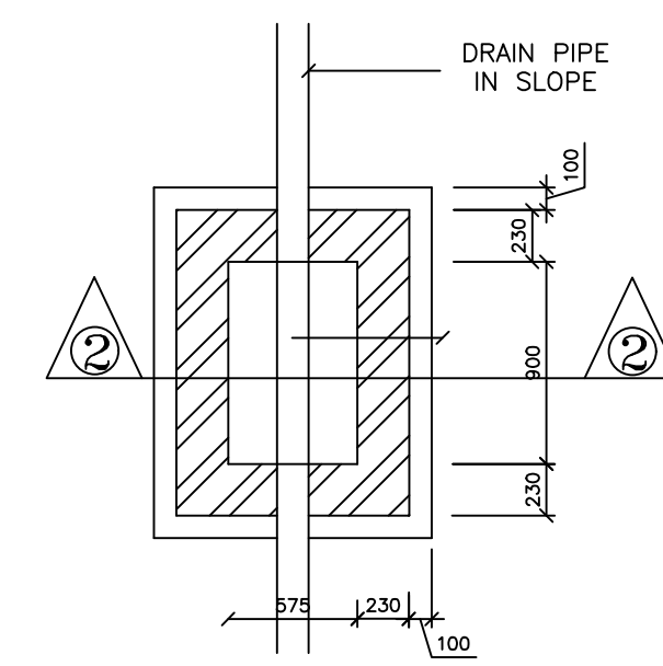
PLAN I.C.DETAILS
