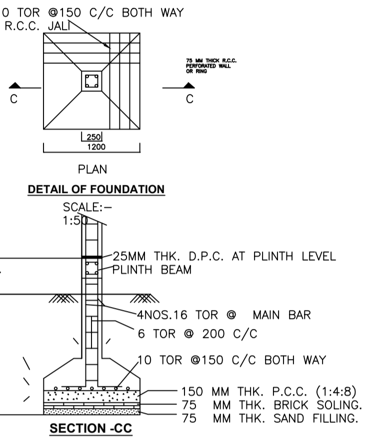
SECTION -CC
