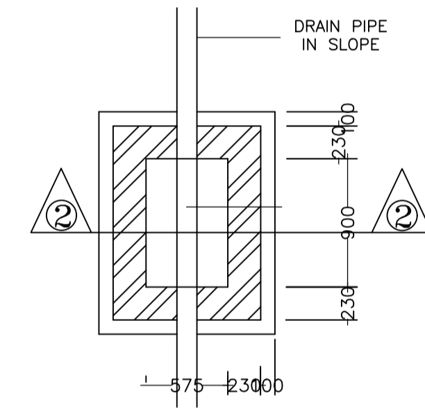
PLAN I.C.DETAILS
