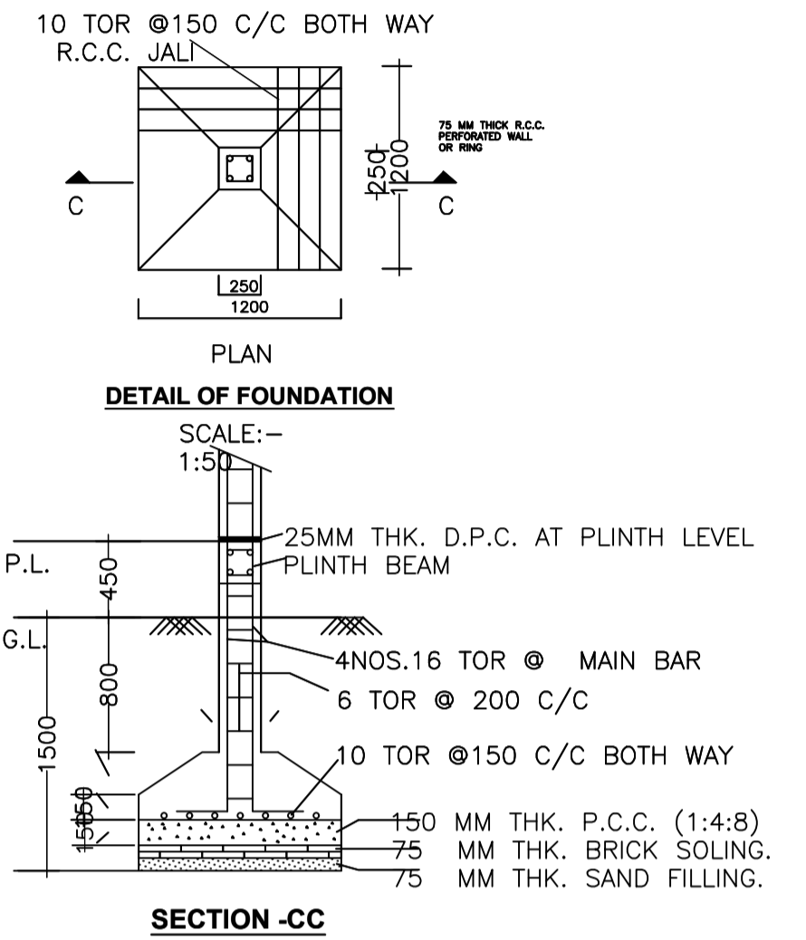
SECTION -CC
