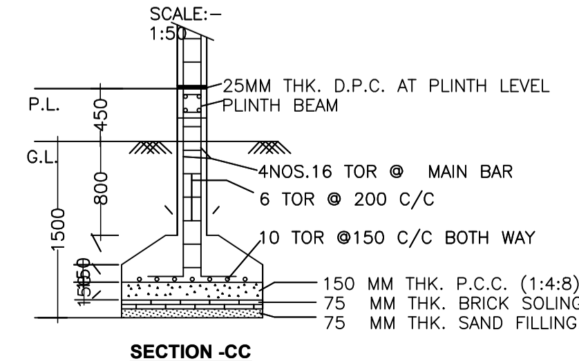
SECTION -CC
