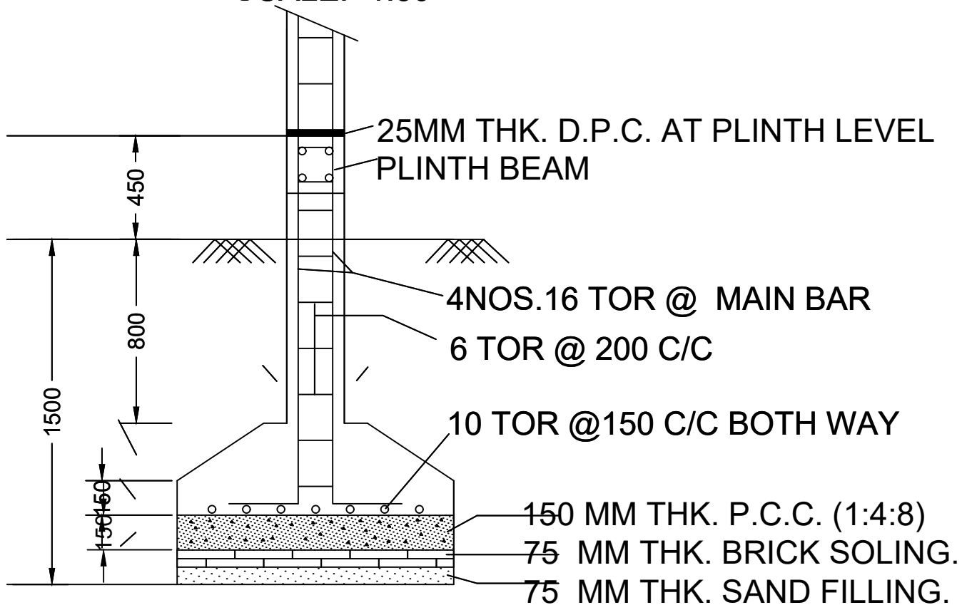
SECTION -CC
