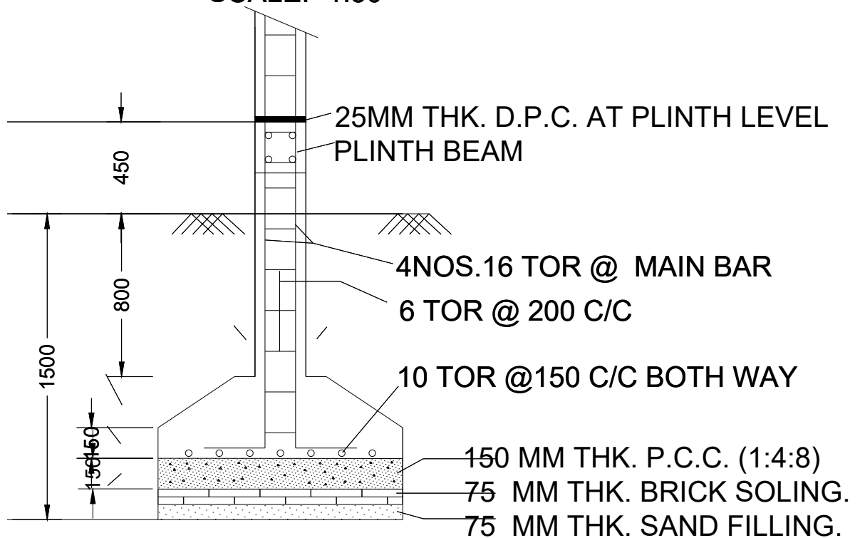
SECTION -CC
