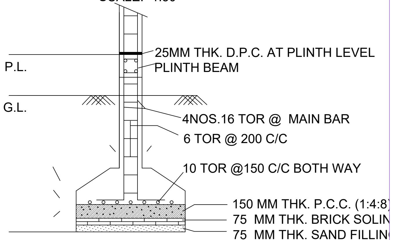
SECTION -CC
