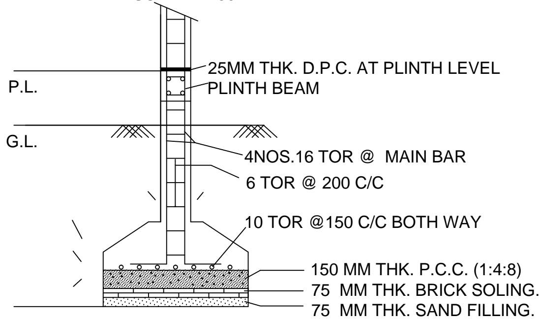
SECTION -CC
