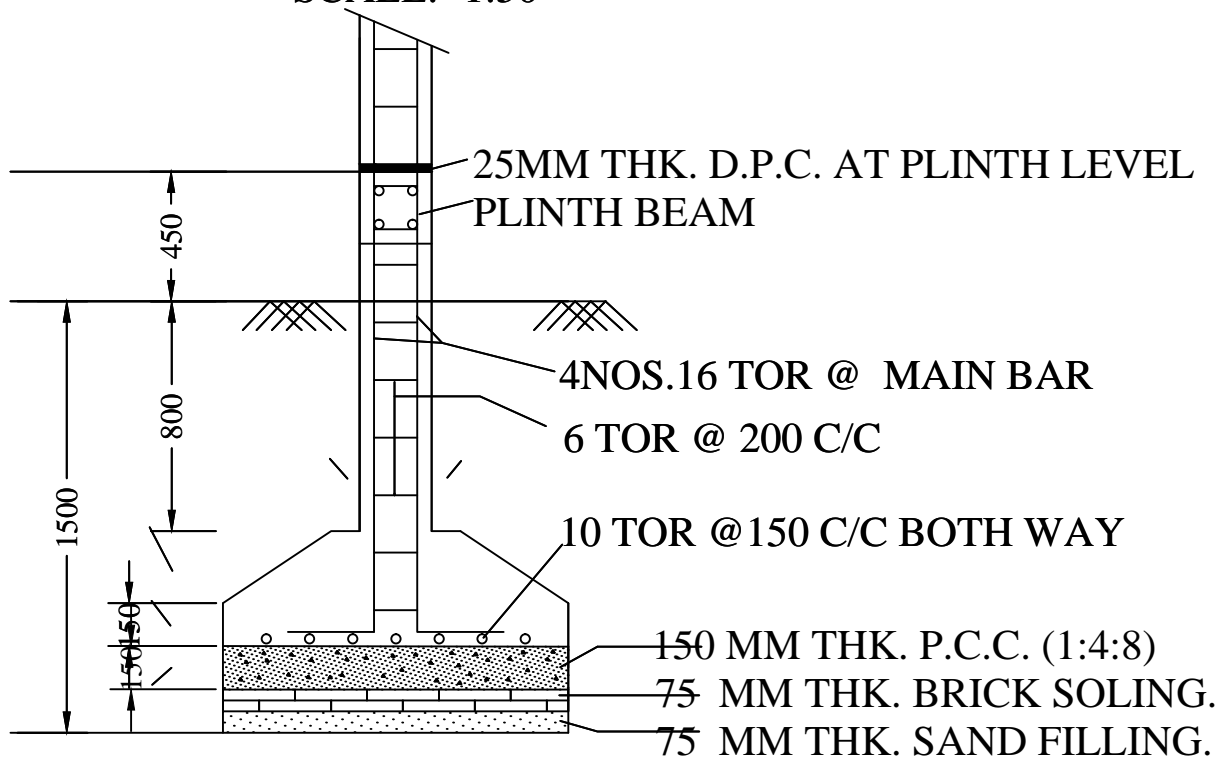
SECTION -CC
