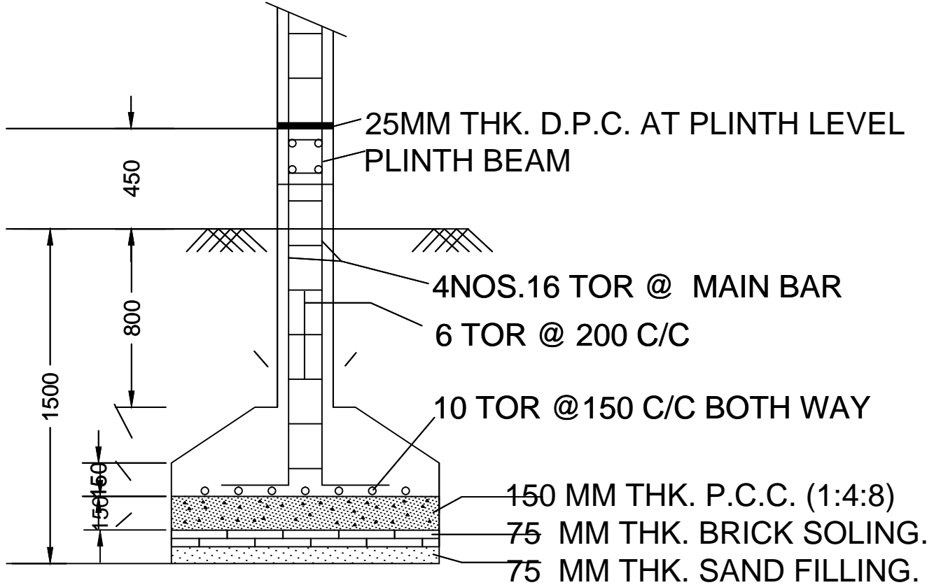
SECTION -CC
