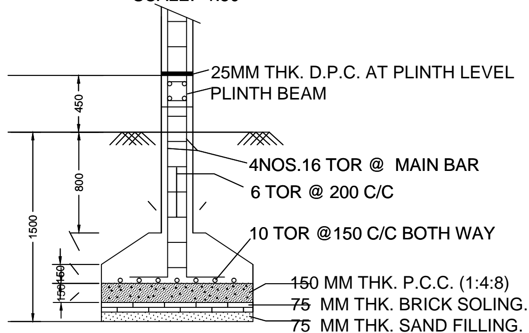
SECTION -CC
