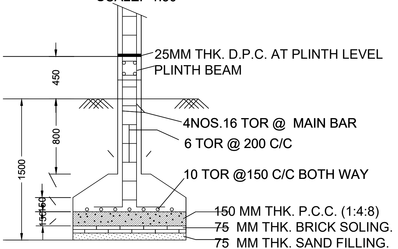
SECTION -CC
