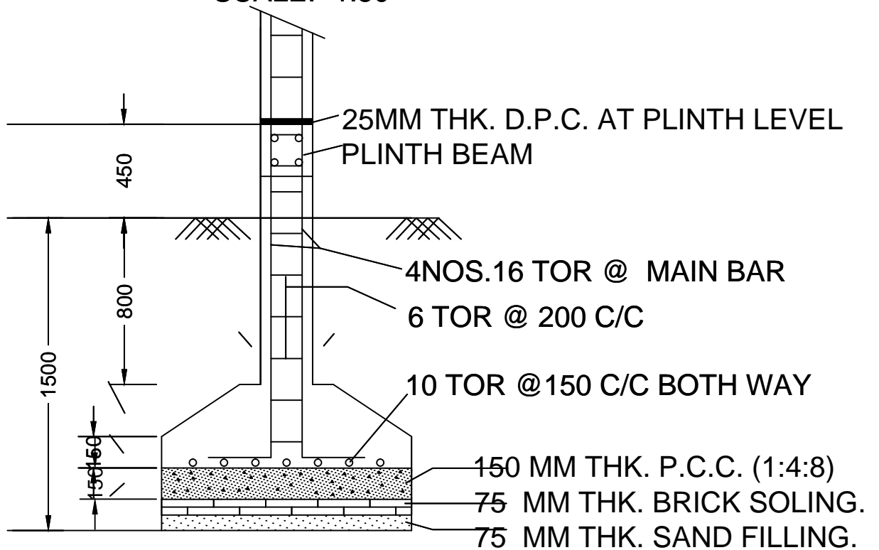
SECTION -CC
