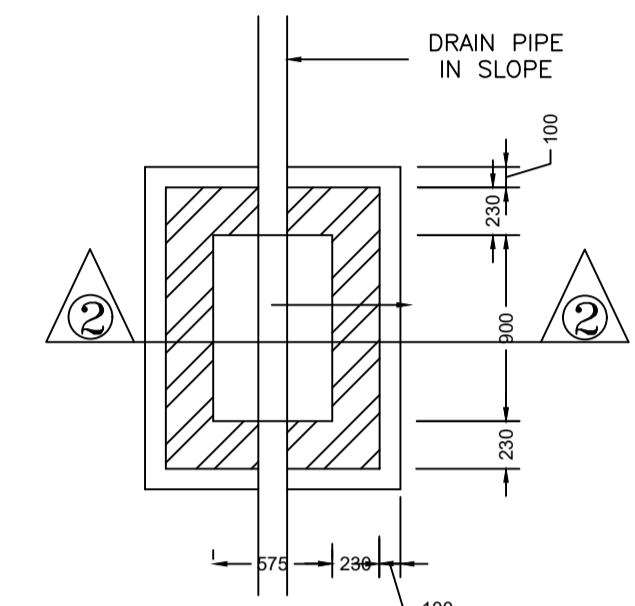
PLAN I.C.DETAILS
