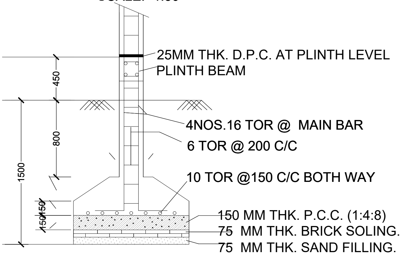
SECTION -CC
