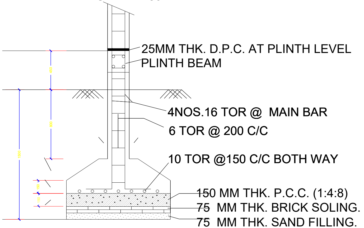
SECTION -CC
