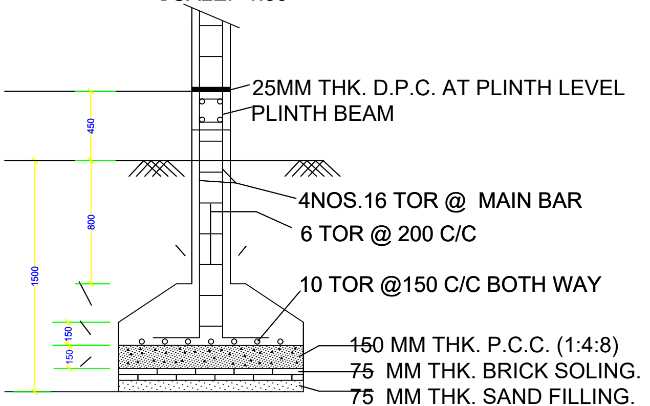
SECTION -CC
