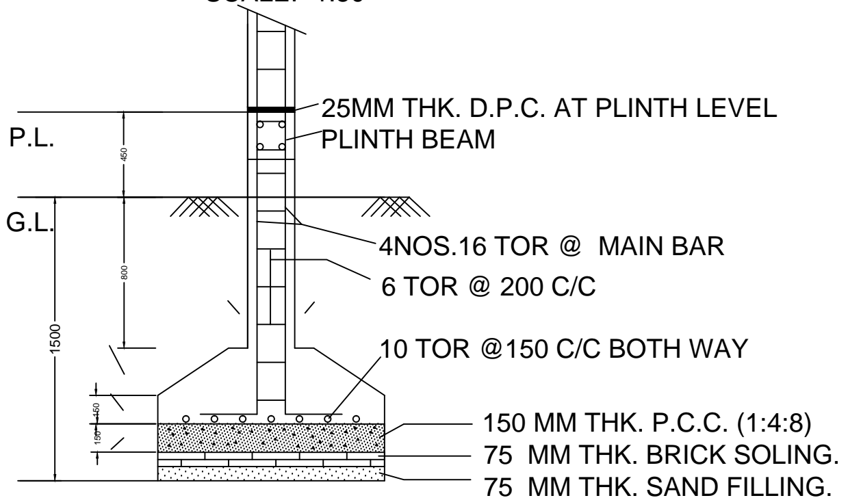
SECTION -CC
