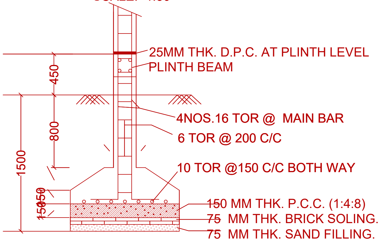
SECTION -CC
