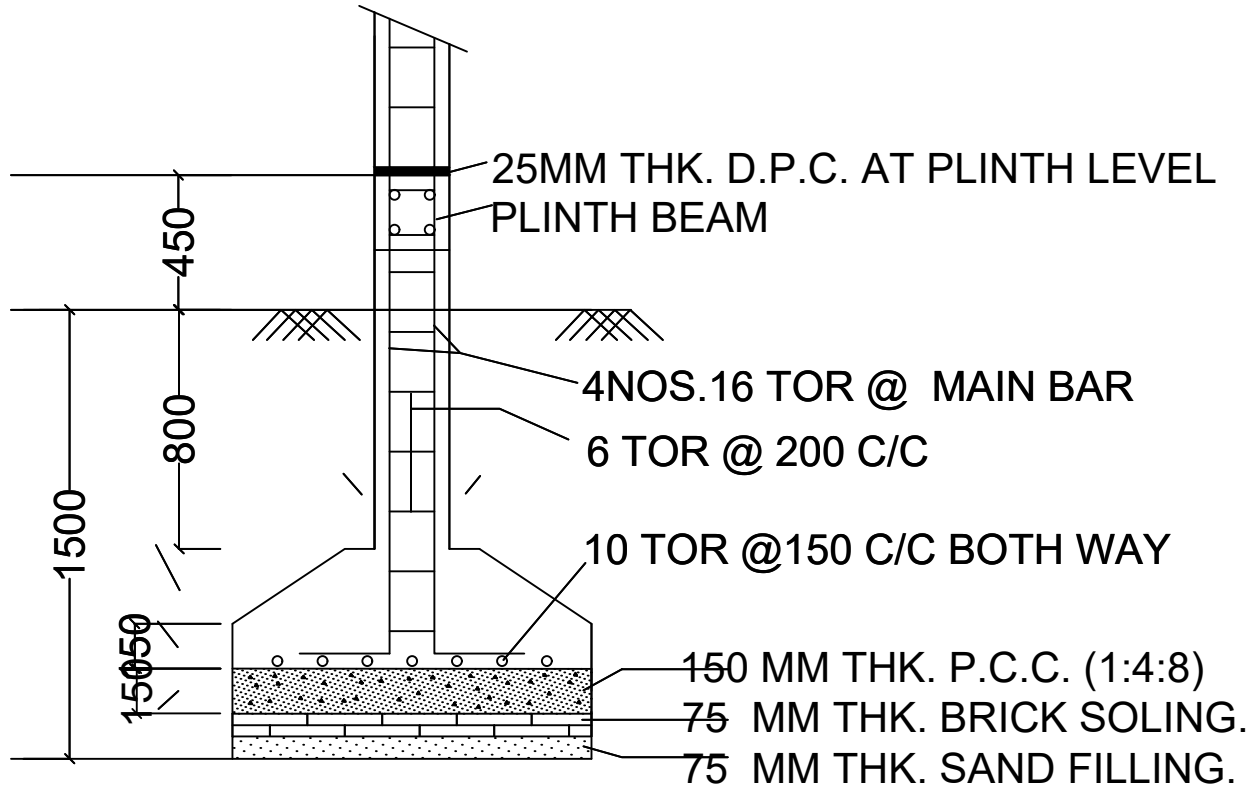
SECTION -CC
