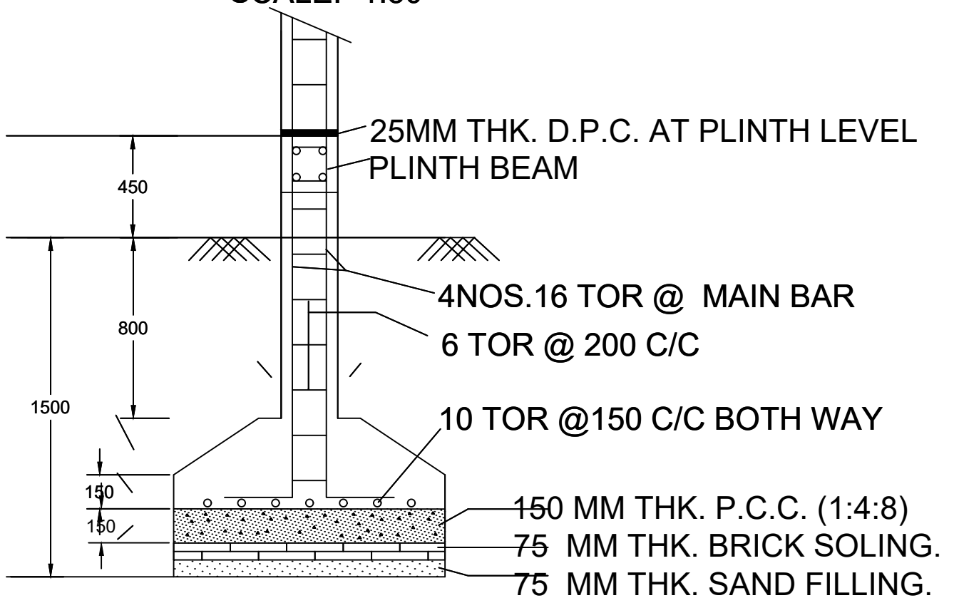
SECTION -CC
