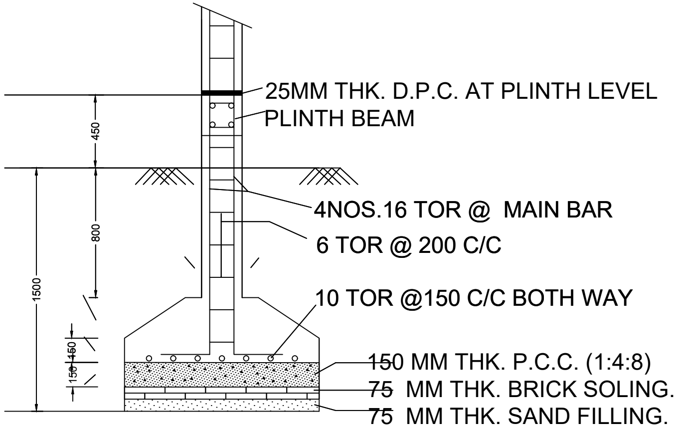
SECTION -CC
