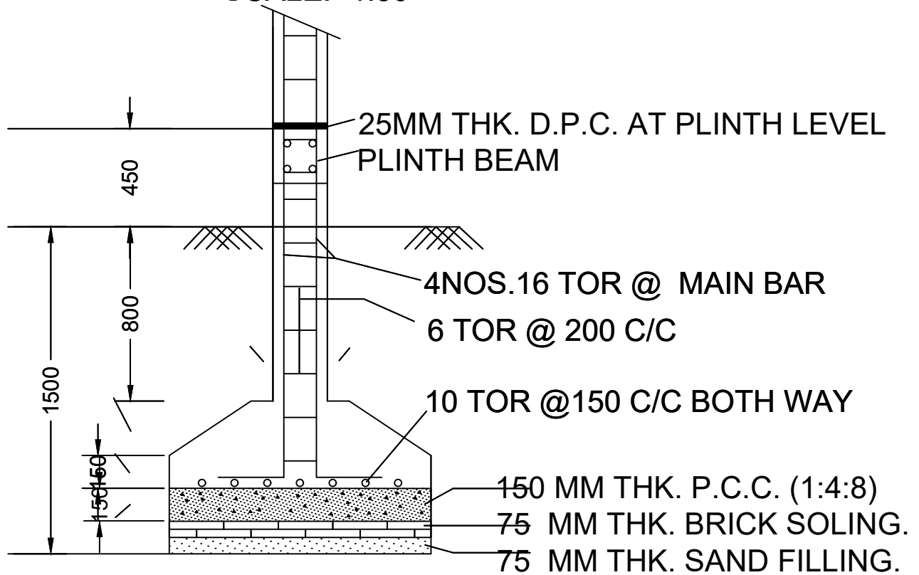
SECTION -CC
