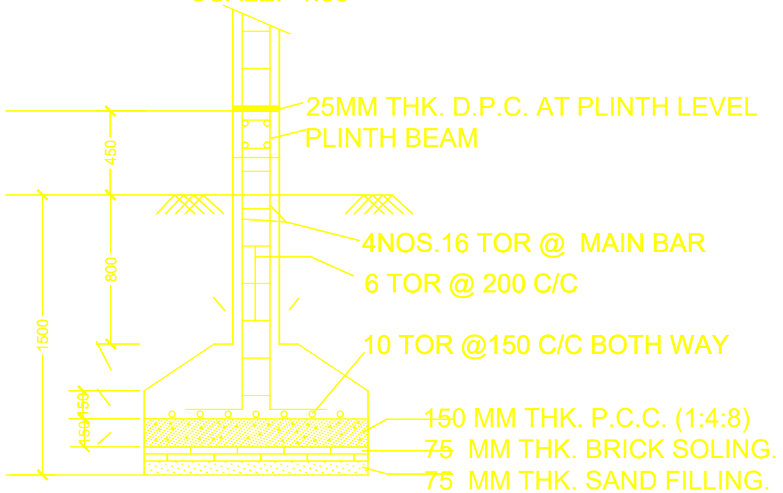
SECTION -CC
