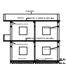
SECTION A-A SCALE: 1:100
