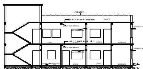
SECTION B-B SCALE: 1:100
