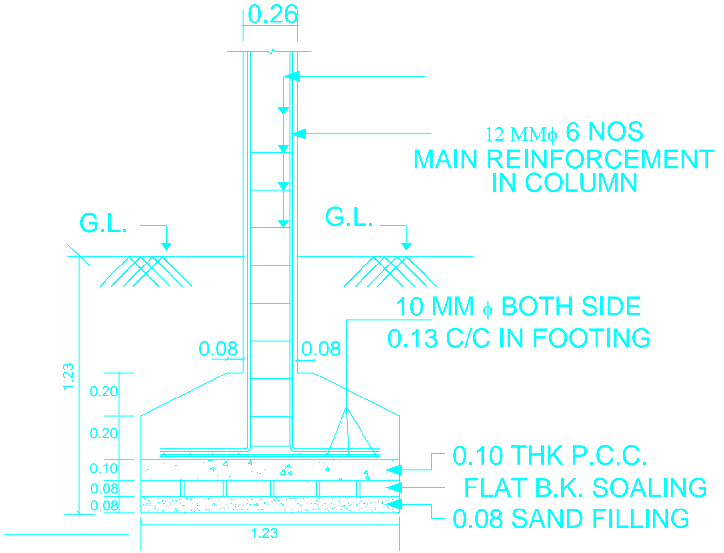
R.C.C. COLUMN
