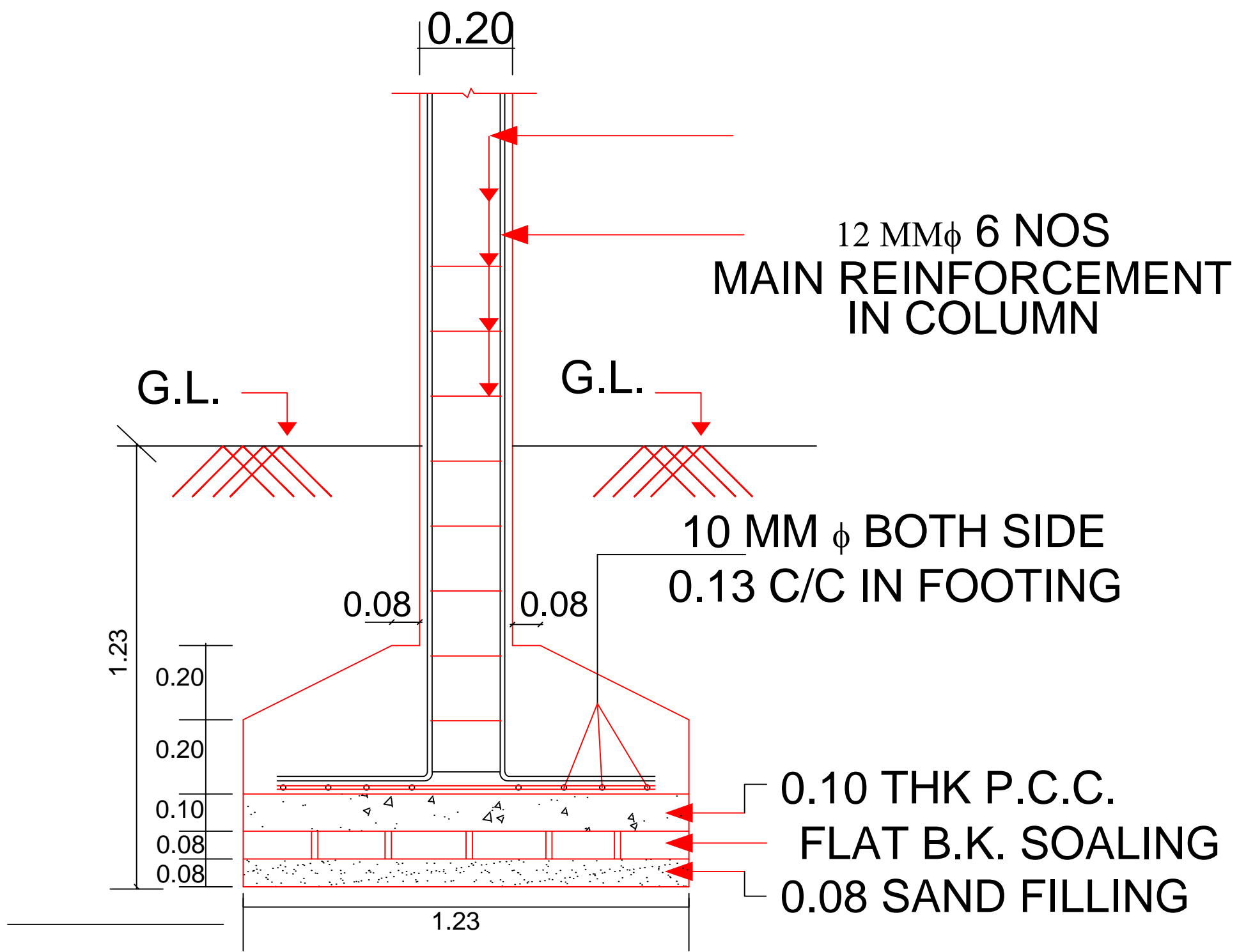
R.C.C. COLUMN FDN.DETAIL
