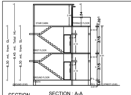
SECTION SECTION : A-A
