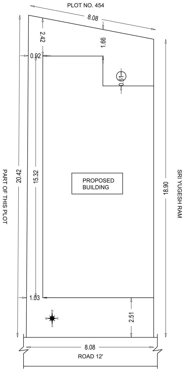
SITE PLAN 1"=8'
