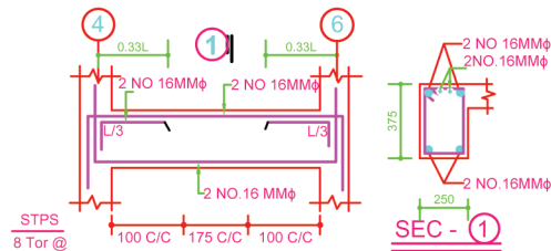
DET. OF R.B.- (250X375)
