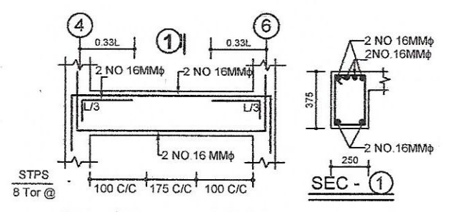
DET. OF R.B.- (250X375)
