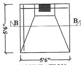
FOUNDATION COL.(10"X15")
