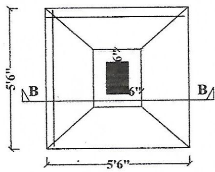
FOUNDATION COL.(10"X15")
