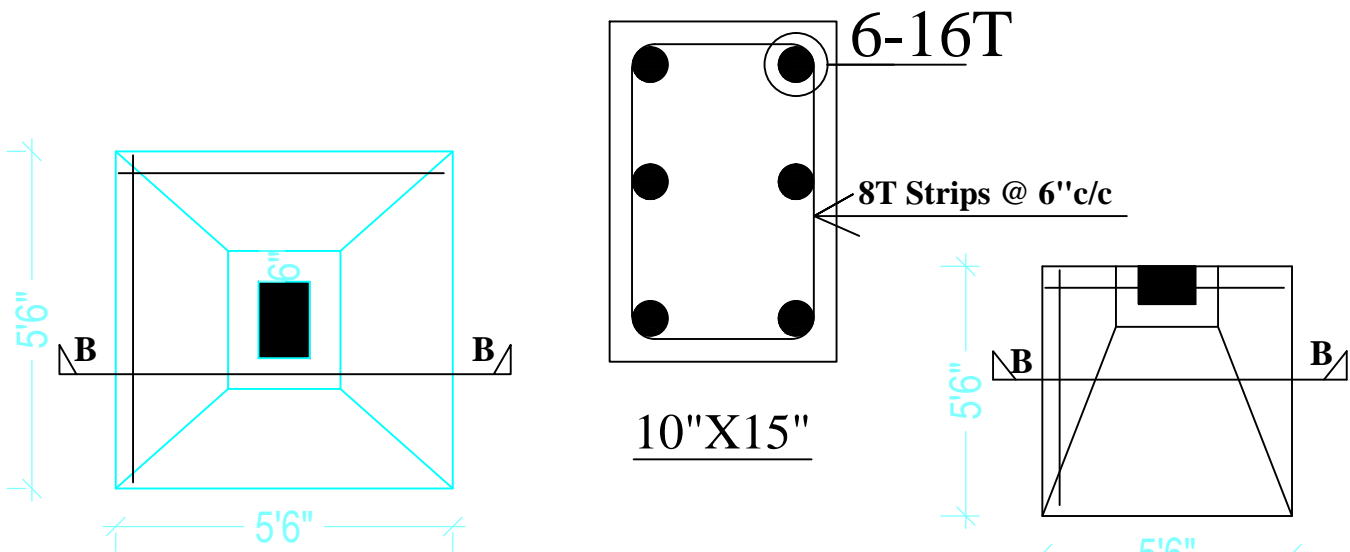
FOUNDATION COL.(10"X15")
