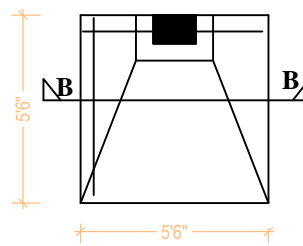
FOUNDATION COL.(10"X15")
