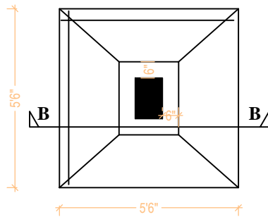
FOUNDATION COL.(10"X15")
