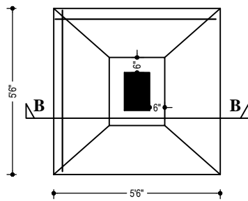
FOUNDATION COL.(10"X15")
