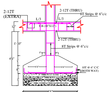
SECTION - D-D
