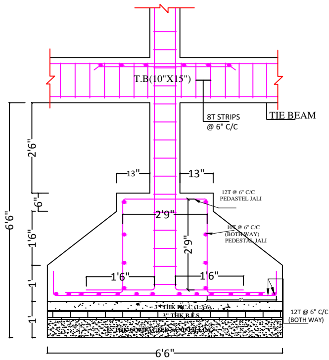
SECTION - A-A C1
