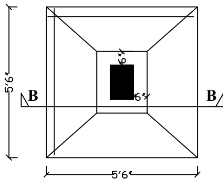
FOUNDATION COL.(10"X15")
