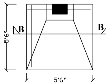
FOUNDATION COL.(10"X15")
