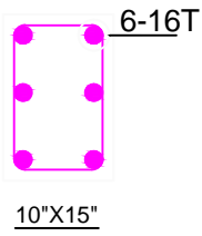
SECTION - D-D
