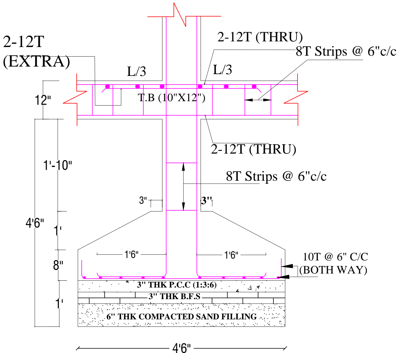
SECTION - D-D
