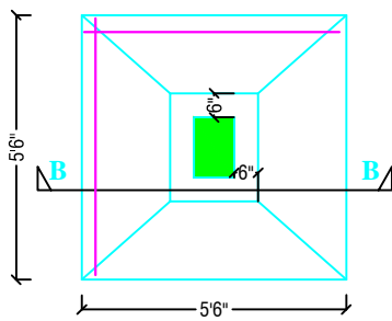
FOUNDATION COL.(10"X15")
