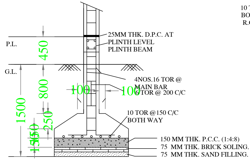
SECTION -CC
