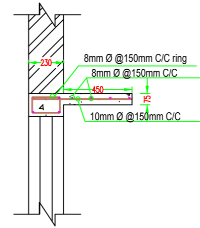
DET. OF R.C.C. CHAJJA
