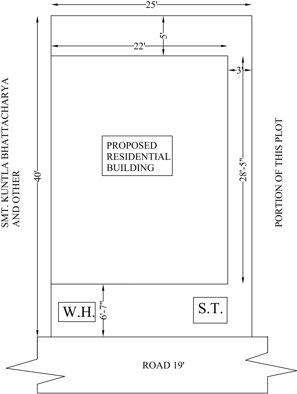
SITE PLAN 1"=8'
