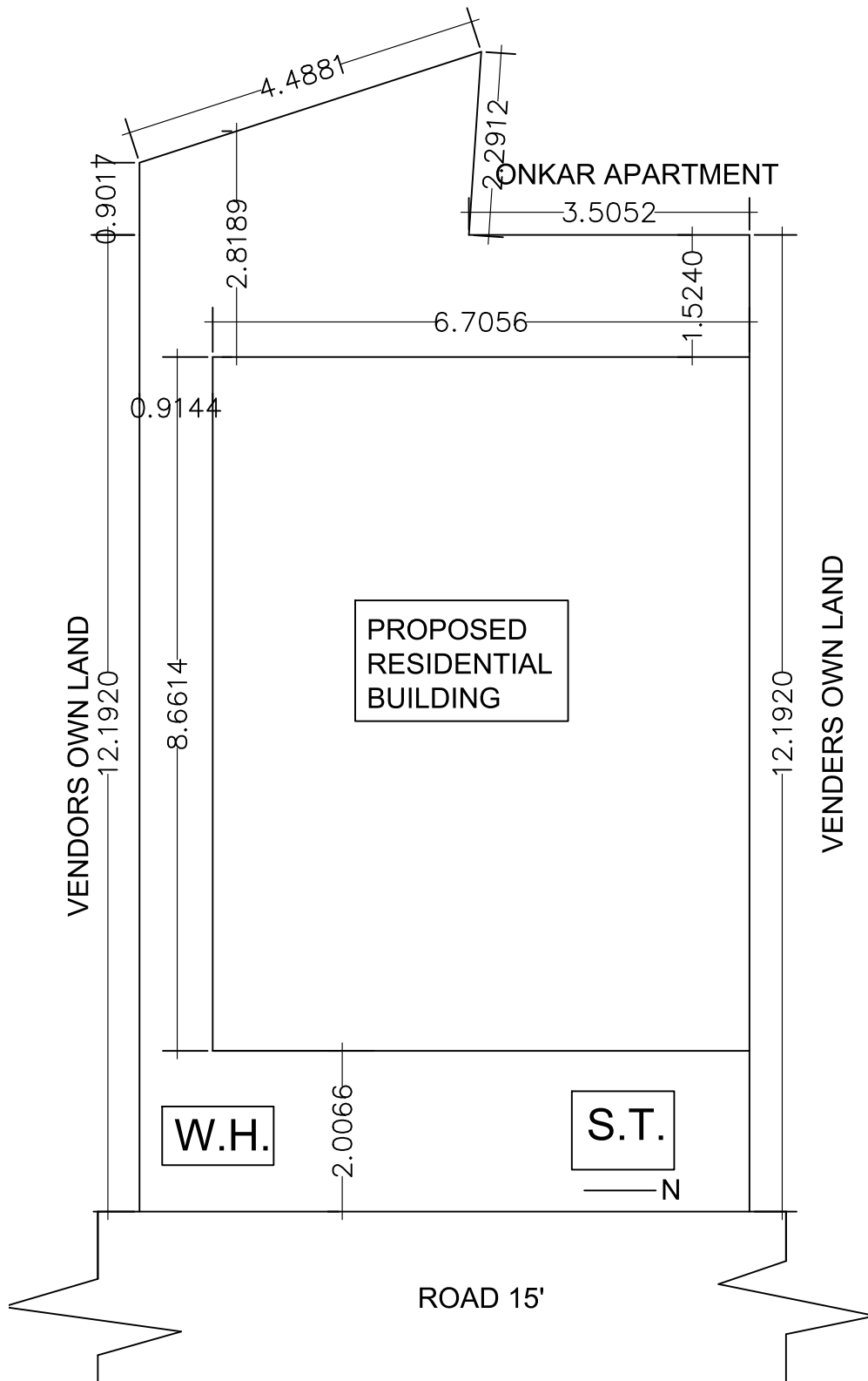
SITE PLAN 1"=8'
